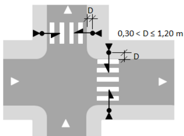
Figura 10.14: Afastamento da botaieira com relação ao meio-fio
