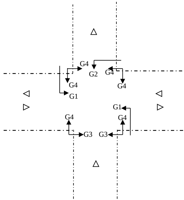
Figura 7.26: Distribuição dos grupos semaforicos
