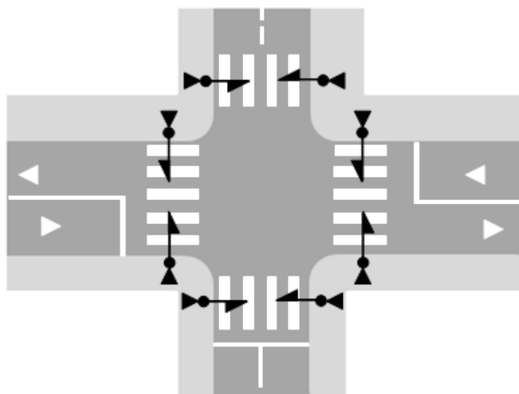
Figura 10.13: Posicionamento da botaieira junto à interseção
